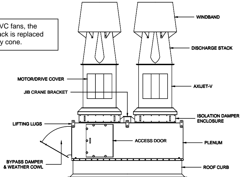
Figure-2. Axijet-V Fan & Plenum Assembly (KVC - Similar)
